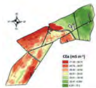
Figura 22 | Exemplo da Condutividade Elétrica Aparente do solo de uma parcela
